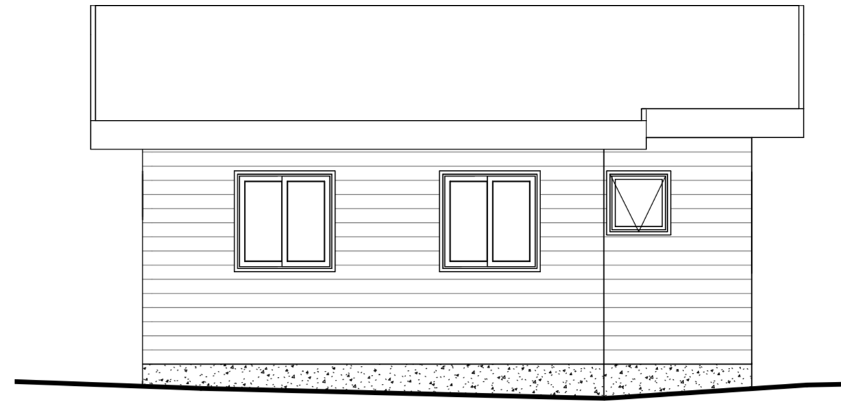
ELEVACIÓN NORTE ESC. 1/50
