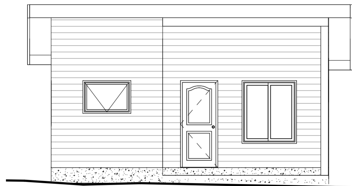
ELEVACIÓN SUR ESC. 1/50
