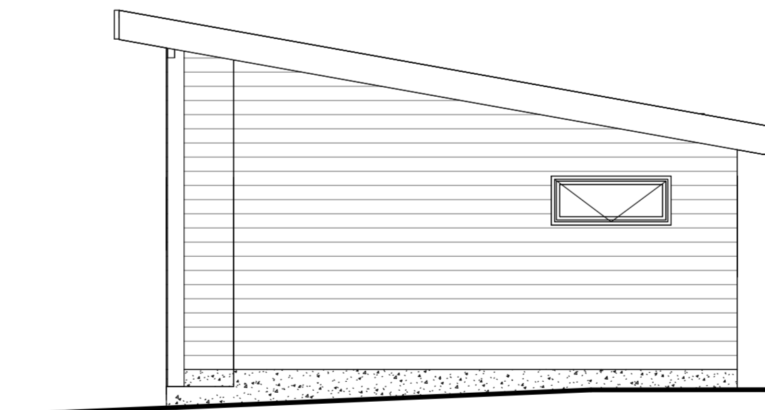
ELEVACIÓN ESTE ESC. 1/50
