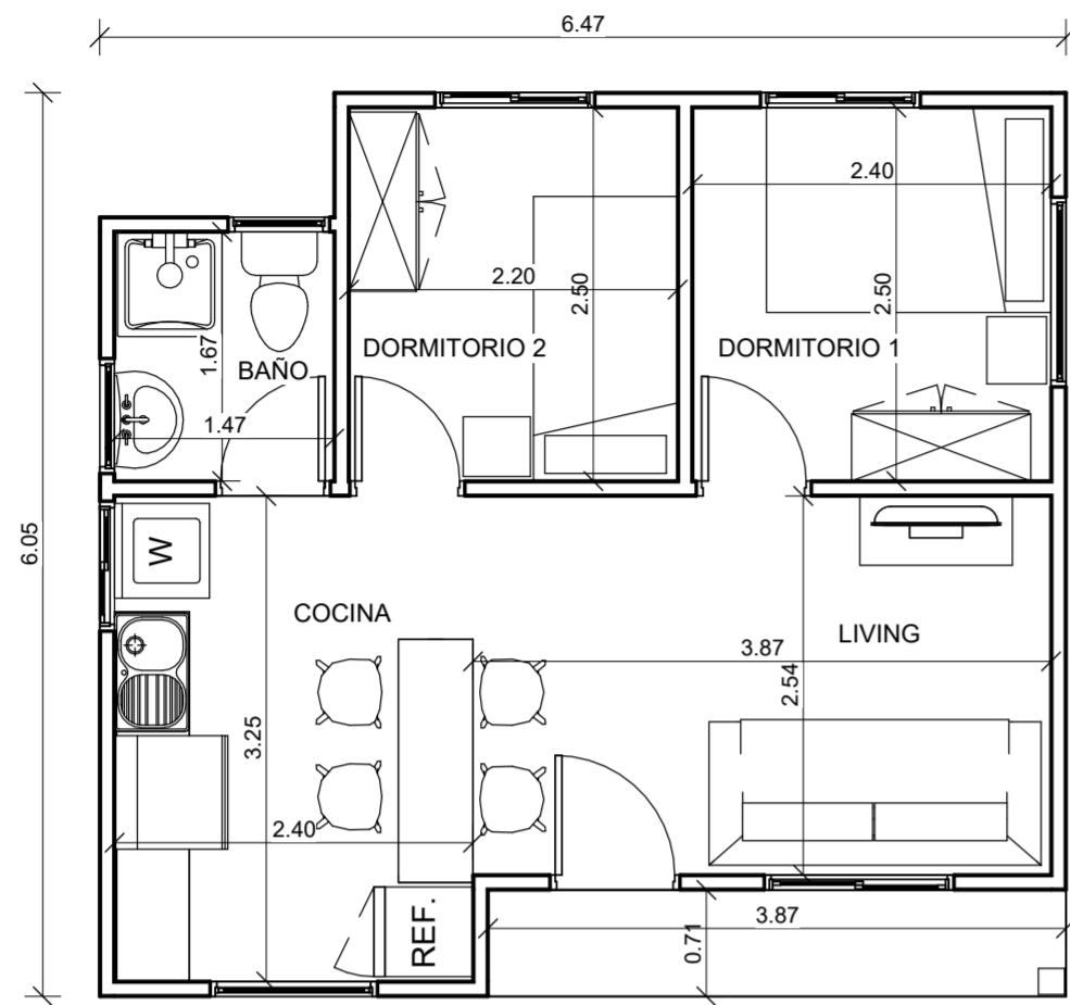
PLANTA DE ARQUITECTURA ESC. 1/50
