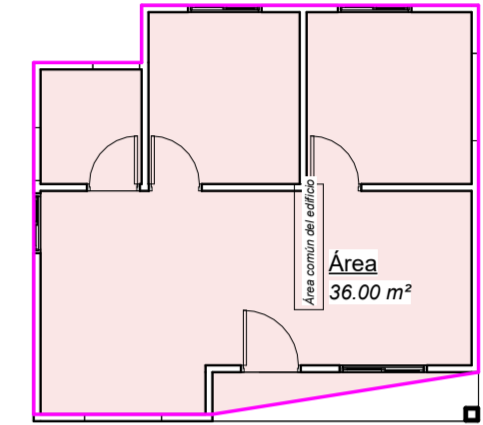
PLANO DE SUPERFICIE ESC. 1/100
